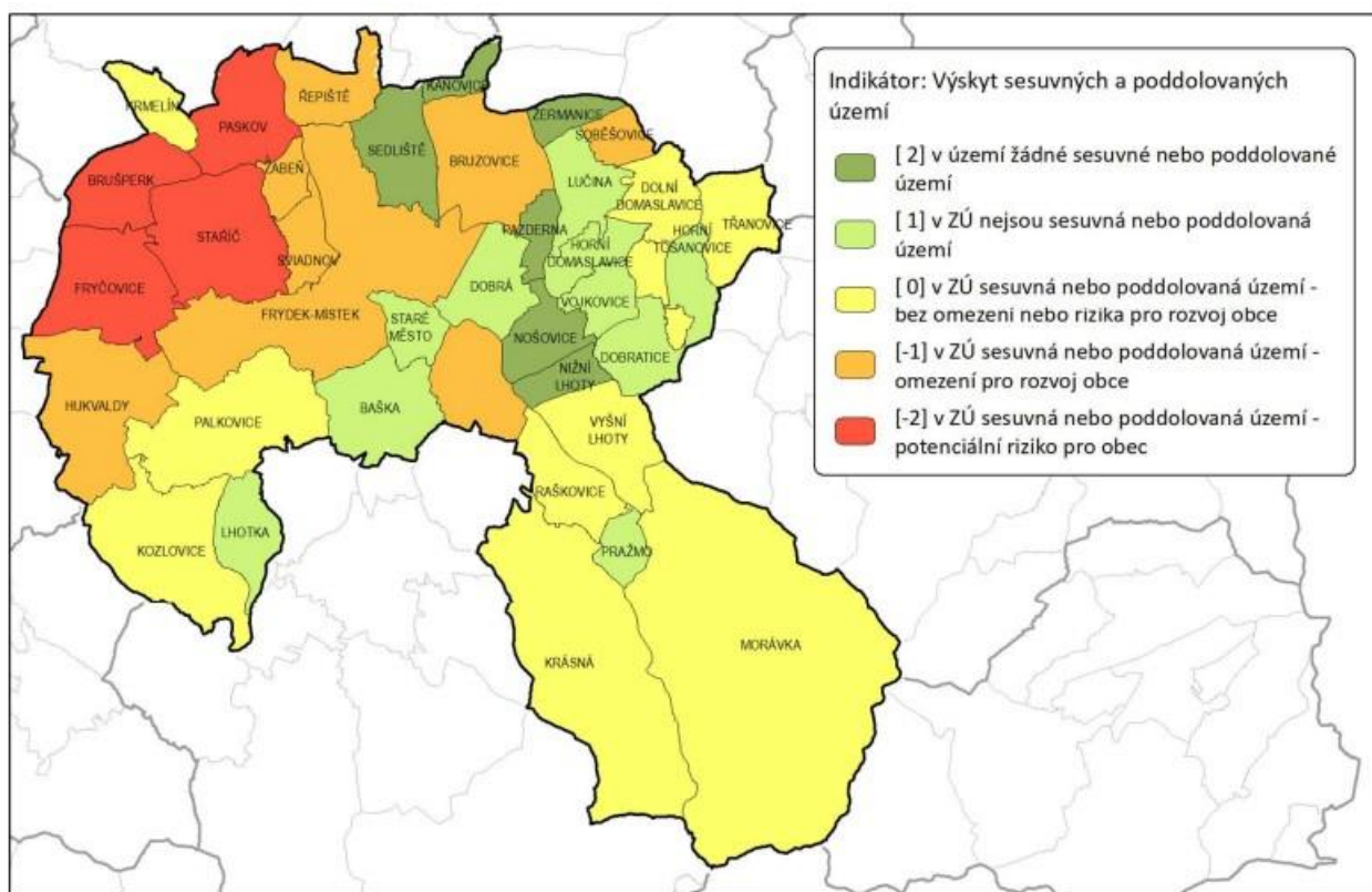
Mapa 9 Výskyt sesuvných a poddolovaných území na území SO ORP Frýdek–Místek
